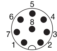
M8 8-polig Stecker/Winkel
