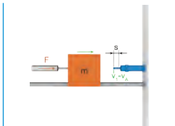
L6. 항상 결합 구동력을 갖는 수평 운동 질량부
